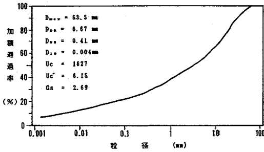
図-6 原位置試験土の粒径加積曲線
