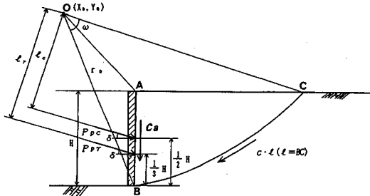
図-2 対数らせん法による受働破壊面
