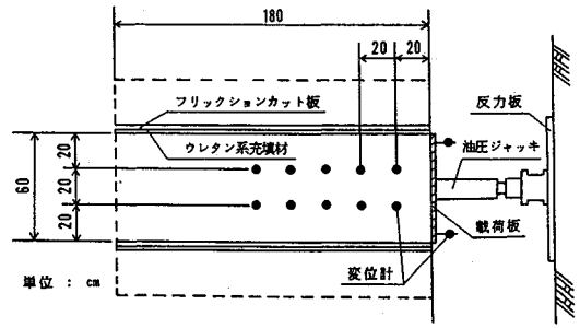
図-3 現場受働土圧型せん断試験の平面図
