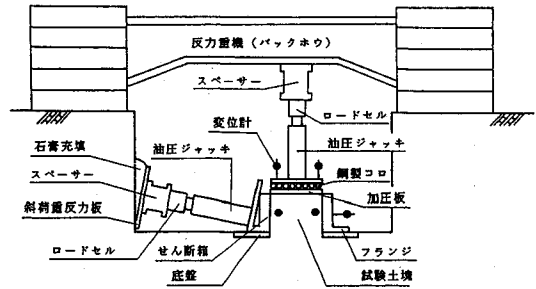
図-15 現場直接せん断試験の試験装置
