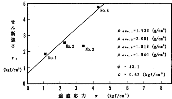
図-16 現場直接せん断試験から求めた \sigma - \tau_f 図
