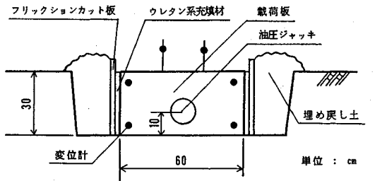
図-5 現場受働土圧型せん断試験の加圧板正面図
