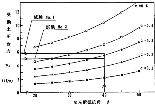
図-13 せん断抵抗角 \phi と受働土圧合力 P_p の関係 ( \delta=3^\circ の場合)
