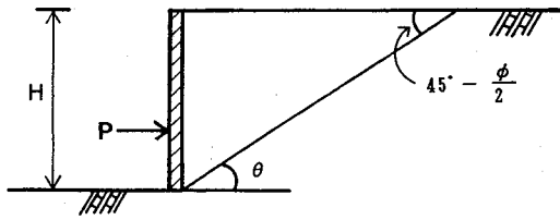
図-1 Rankineの受働土圧論による破壊面とせん断抵抗角φの関係
