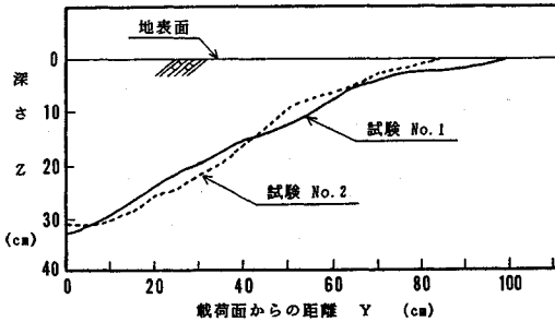
図一〇 縦断面上の破壊形状 (X=20~40 cm の平均)
