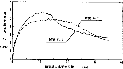
図-7 水平変位量と受働土圧合力 ( P_p ) の関係
