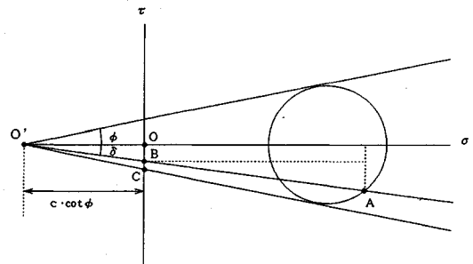
付図一1 壁面の応力状態を示すモール円
