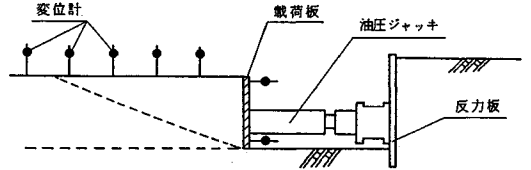
図-4 現場受働土圧型せん断試験の縦断面図
