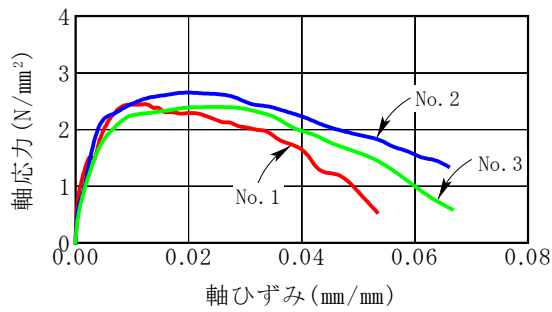
図-2 応力～ひずみ曲線(実験結果)
