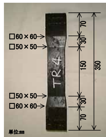
図-1 供試体形状
